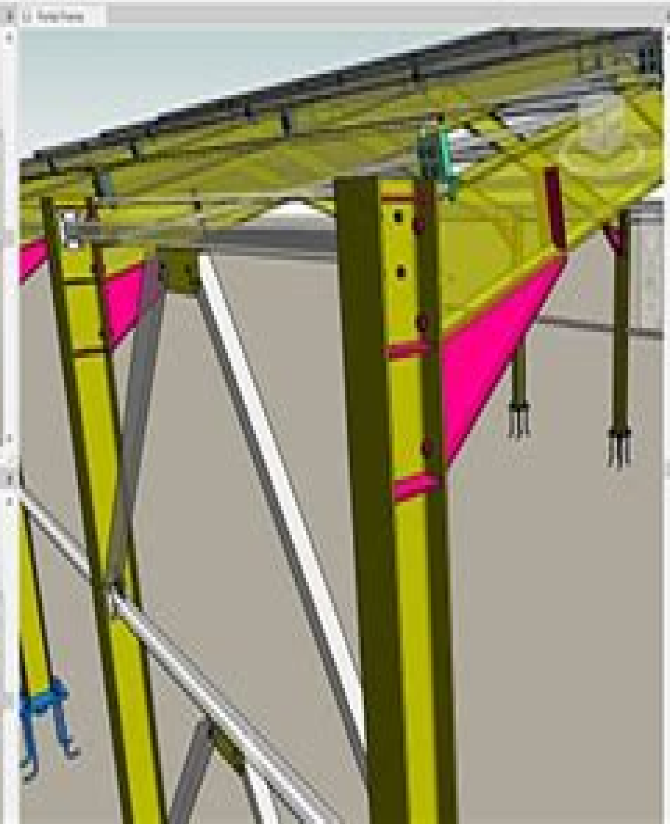
Fig. 12: Frame
