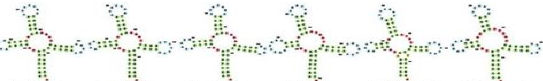
tRNA - Glu
